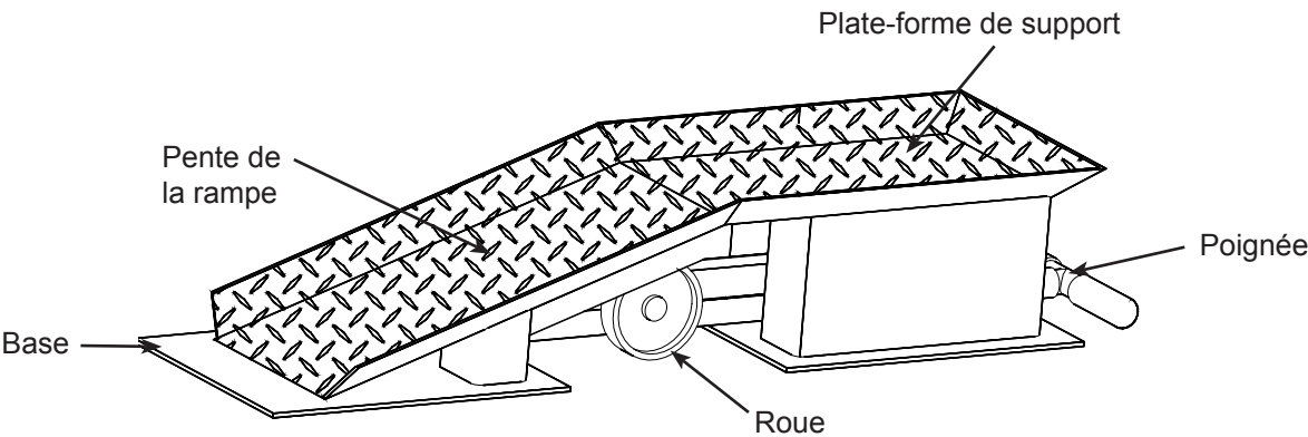
Figure 1 : Composants d'une rampe pour camion
