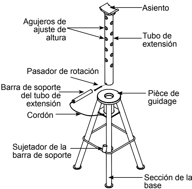
Figure 1 : Composantes de los modelos 32105B y 32107B
